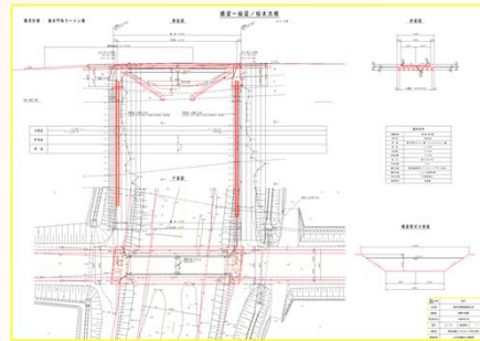
橋梁一般図
