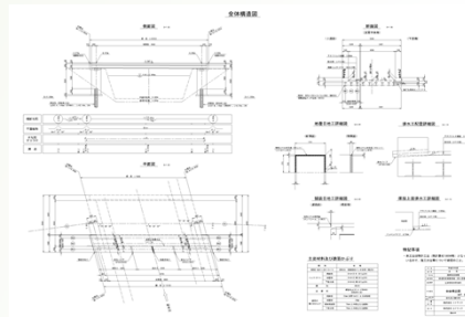
橋梁一般図
