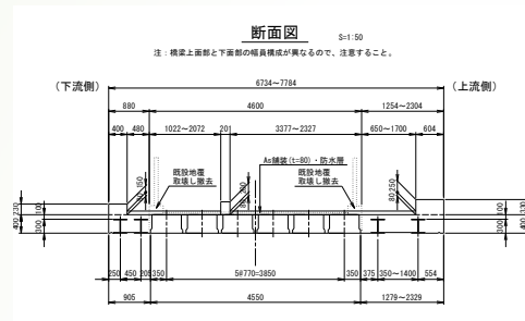
橋梁一般図
