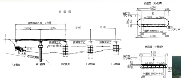
橋梁一般図
