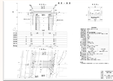
橋梁一般図
