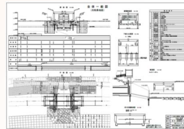
橋梁一般図
