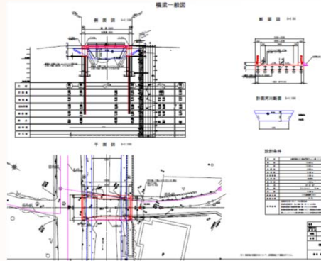
橋梁一般図
