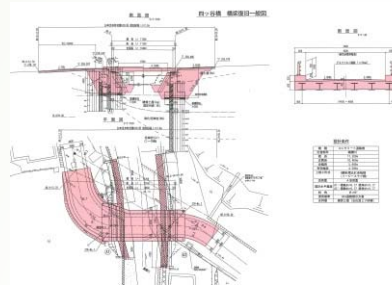
橋梁一般図
