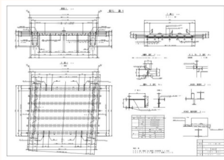
橋梁一般図
