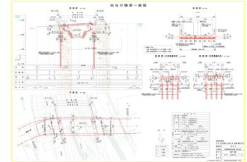
橋梁一般図
