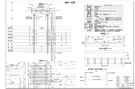
橋梁一般図
