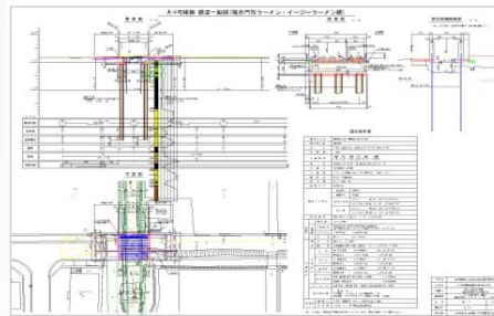
橋梁一般図
