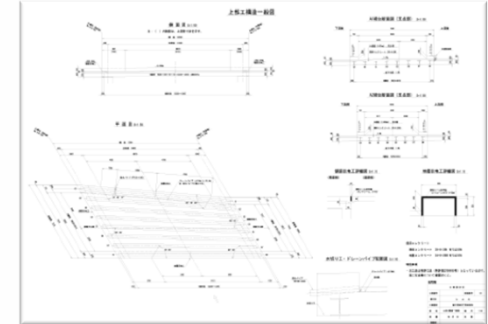
橋梁一般図
