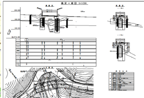
橋梁一般図
