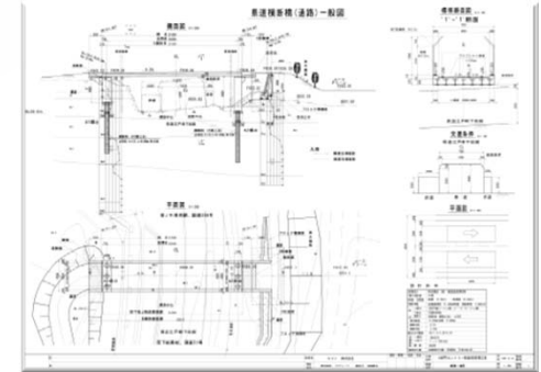
橋梁一般図
